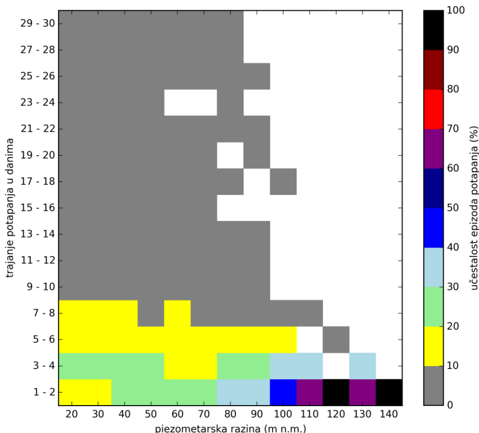
2.19. Učestalost epizoda potapanja podzemnog prostora različitog trajanja za pojedine visinske klase na piezometru O9. Niže visine od najniže koja je prikazana na grafu su stalno potopljene.
