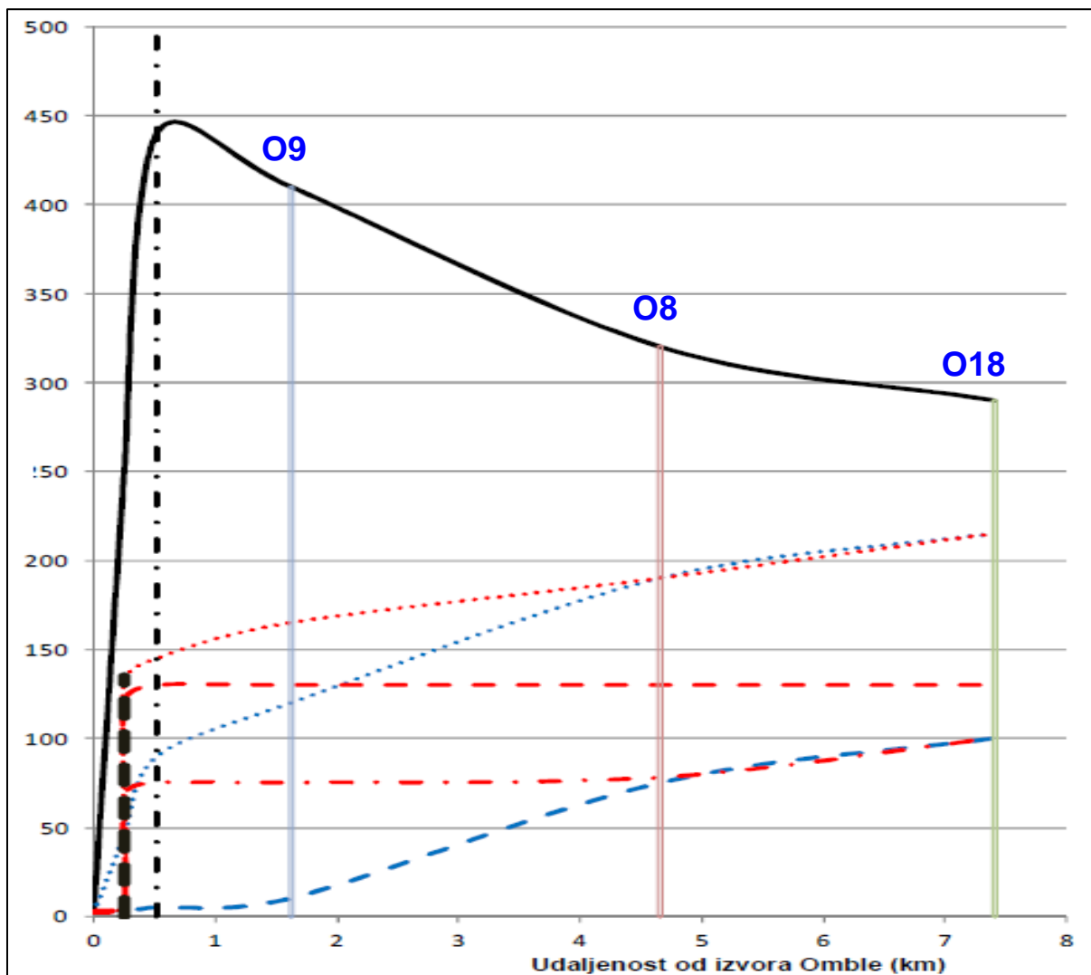
Slika 2.12. Razine podzemne vode u zaleđu Omble prije i nakon izvedbe injekcijske zavjese (preuzeto iz elaborata: PLAN UPRAVLJANJA BIORAZNOLIKOŠĆU, Clegg M, Palmer T. & Beaton S., 2013).
