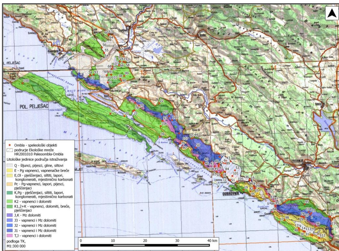
Slika 3.1. Izrez iz listova geoloških karata M 1: 100 000 (OGK Dubrovnik, Ston, Trebinje, Metković, Korčula, Ploče) s prikazanim litološkim jedinicama na širem području istraživanja i lokacijama špiljskih objekata koji su bili predmet istraživanja u ovom projektu (podloga TK M 1: 300 000).
