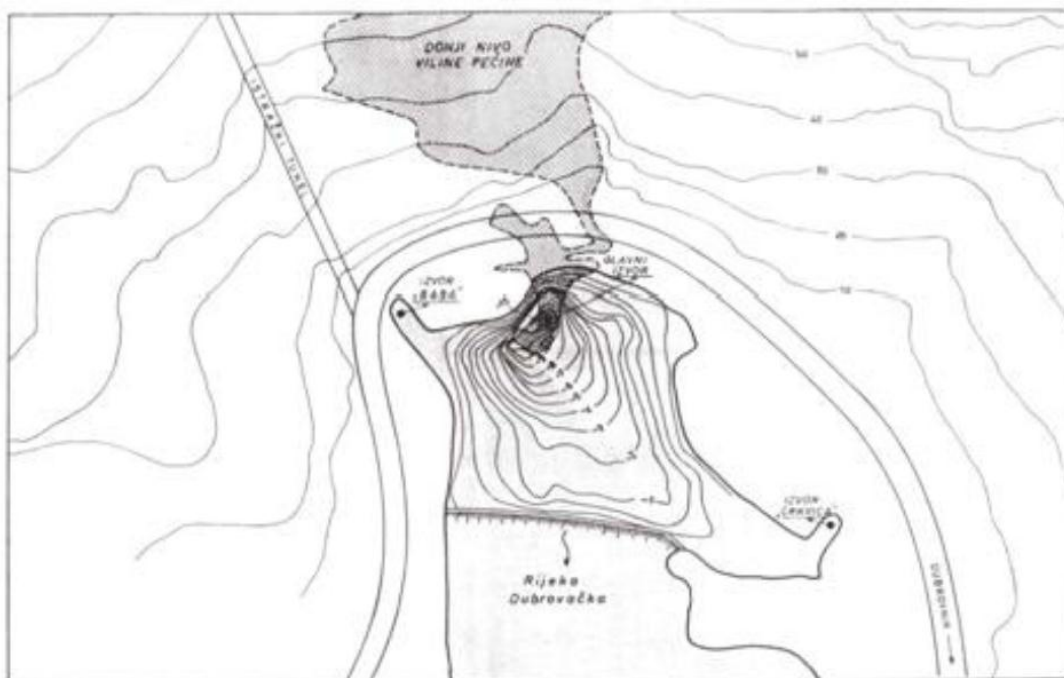
Slika 2.6. Tri zone koncentriranog istjecanja izvorišta Ombla: Glavni izvor, Babe i Crkvice (preuzeto iz elaborata HE OMBLA - Rekapitulacija rezultata istražnih radova i Program mjera zaštite okoliša prije početka i tijekom gradnje hidroelektrane, R. Buljan 2008.).
