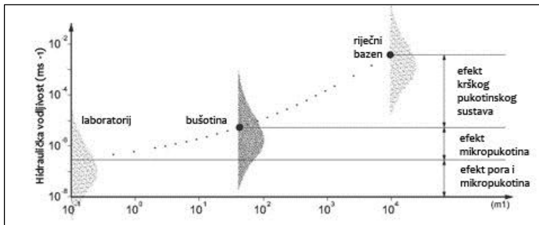
Slika 1.4. Shematski prikaz utjecaja mjerila na hidrauličku vodljivost u kršu (KIRALY, 1975).
